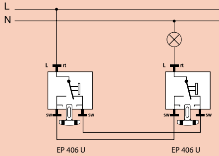
Включение освещения из двух мест
